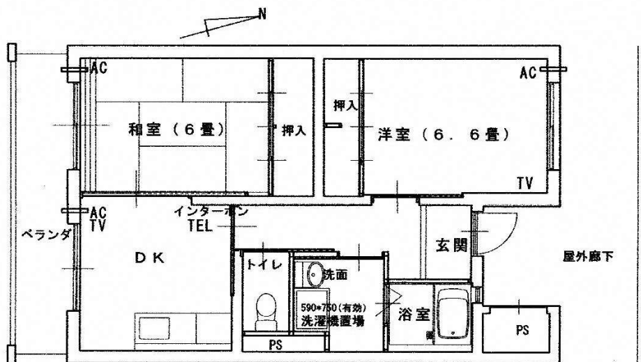
大黒1番館306号室見取図
