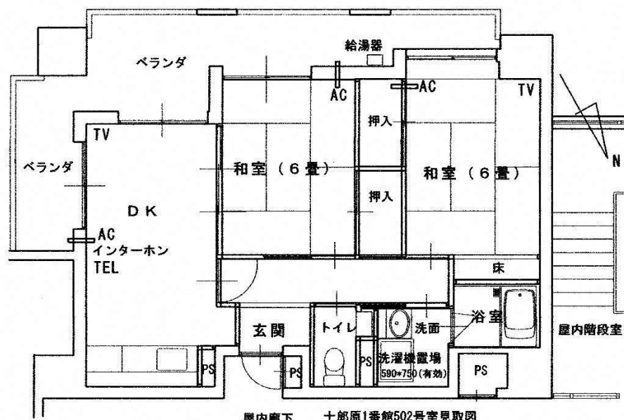
【間取り図】
