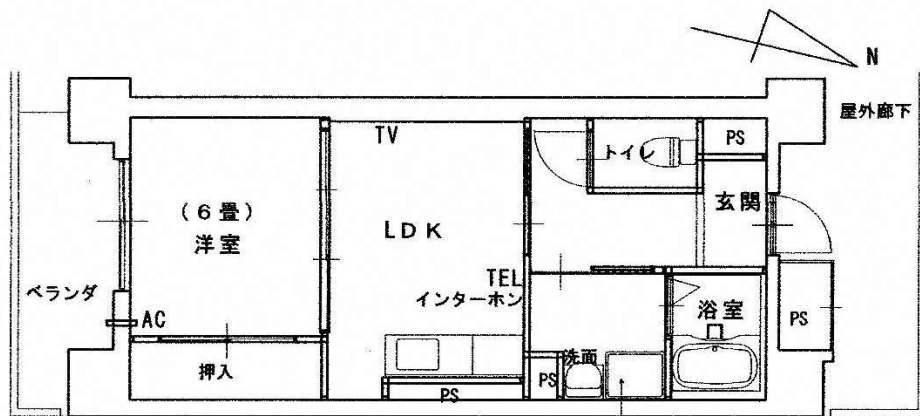
新田5番館401号室見取図
