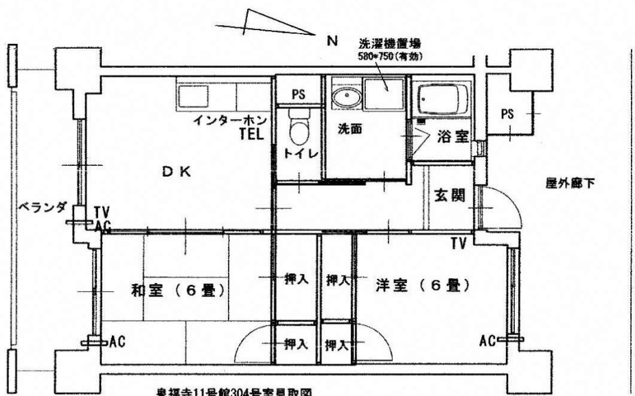
【間取り図】
