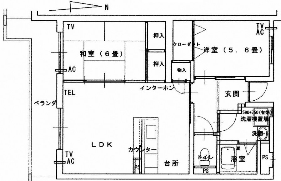
黒石D棟105号室見取図
