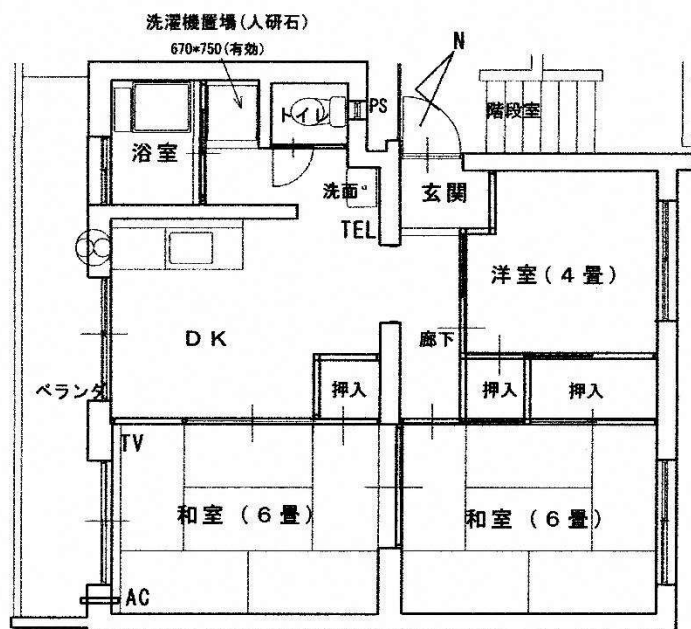
三浦A棟146号室見取図
