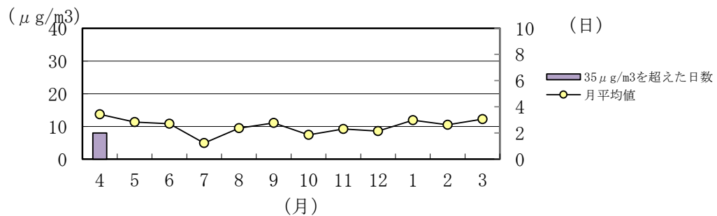
図 7-3 吉井測定局の微小粒子状物質（PM 2.5 ）の月別測定結果
