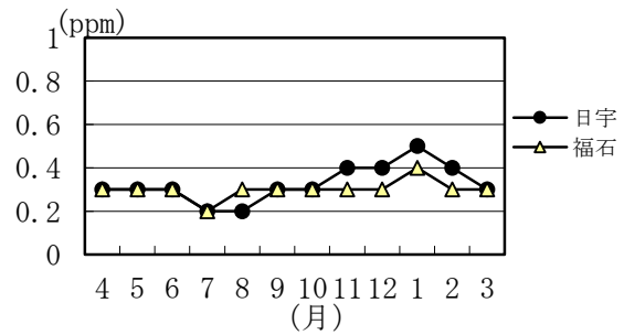
図 6-2 非メタン炭化水素およびメタンの月別測定結果（月平均値）
