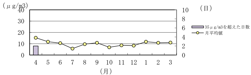
図 7-2 大塔測定局の微小粒子状物質（PM 2.5 ）の月別測定結果
