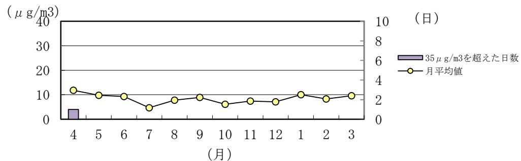
図 7-3 吉井測定局の微小粒子状物質（PM 2.5 ）の月別測定結果
