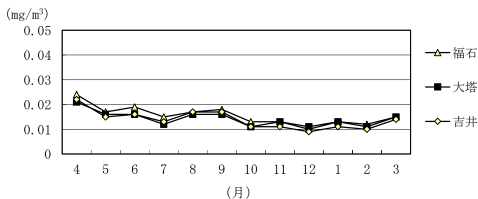
図 2 - 2 浮遊粒子状物質の月別測定結果（月平均値）
