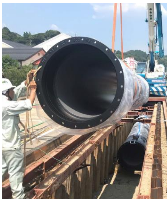
(撮影) 広田水系基幹管路更新事業(φ1000mm工区)
