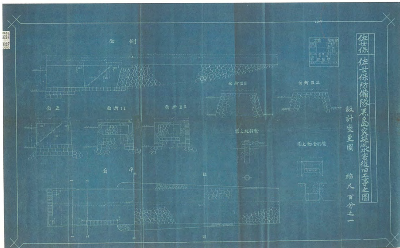
第 100 図 黒島名切突堤復旧工事図面
