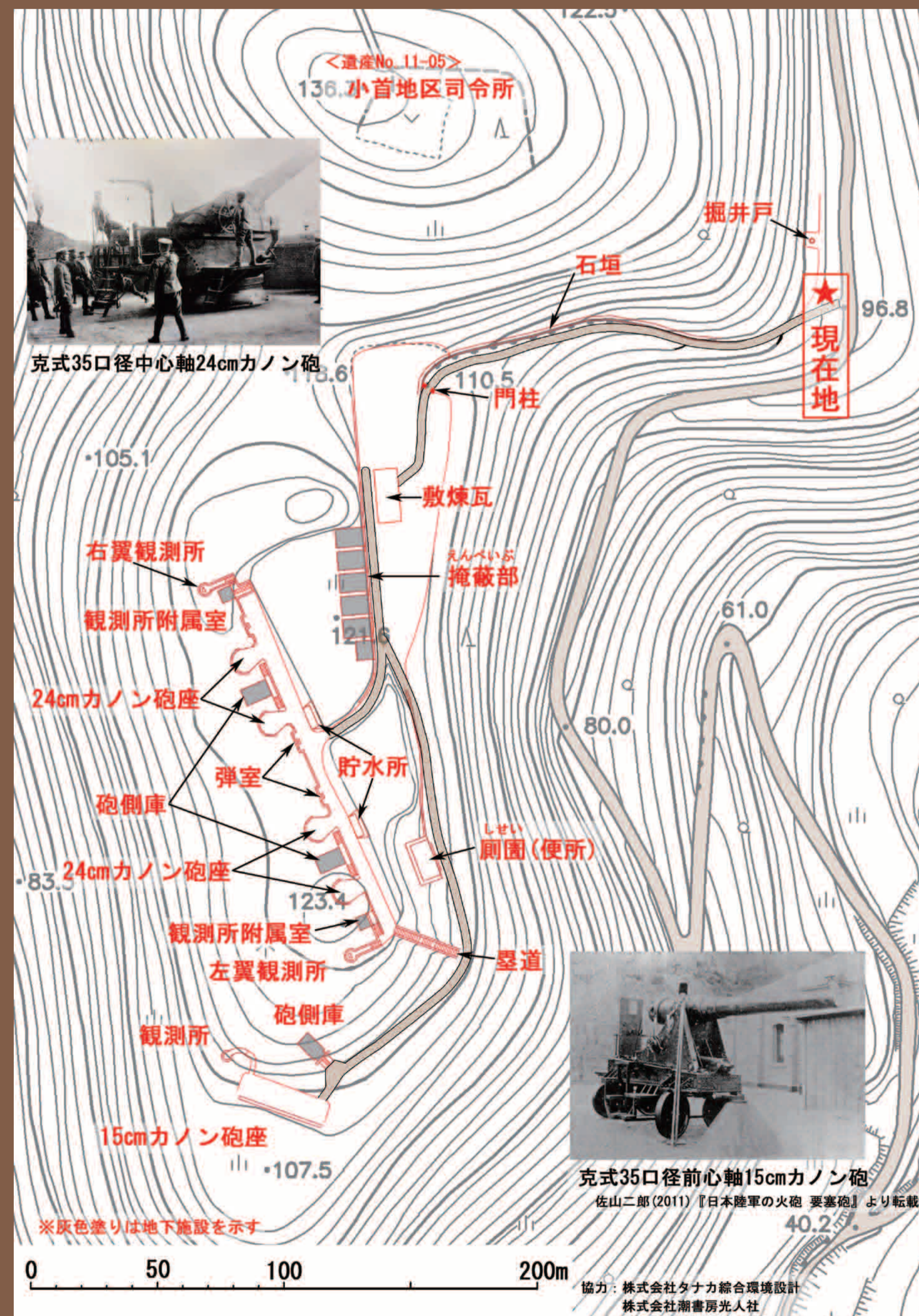
小首堡塁遺構配置図
