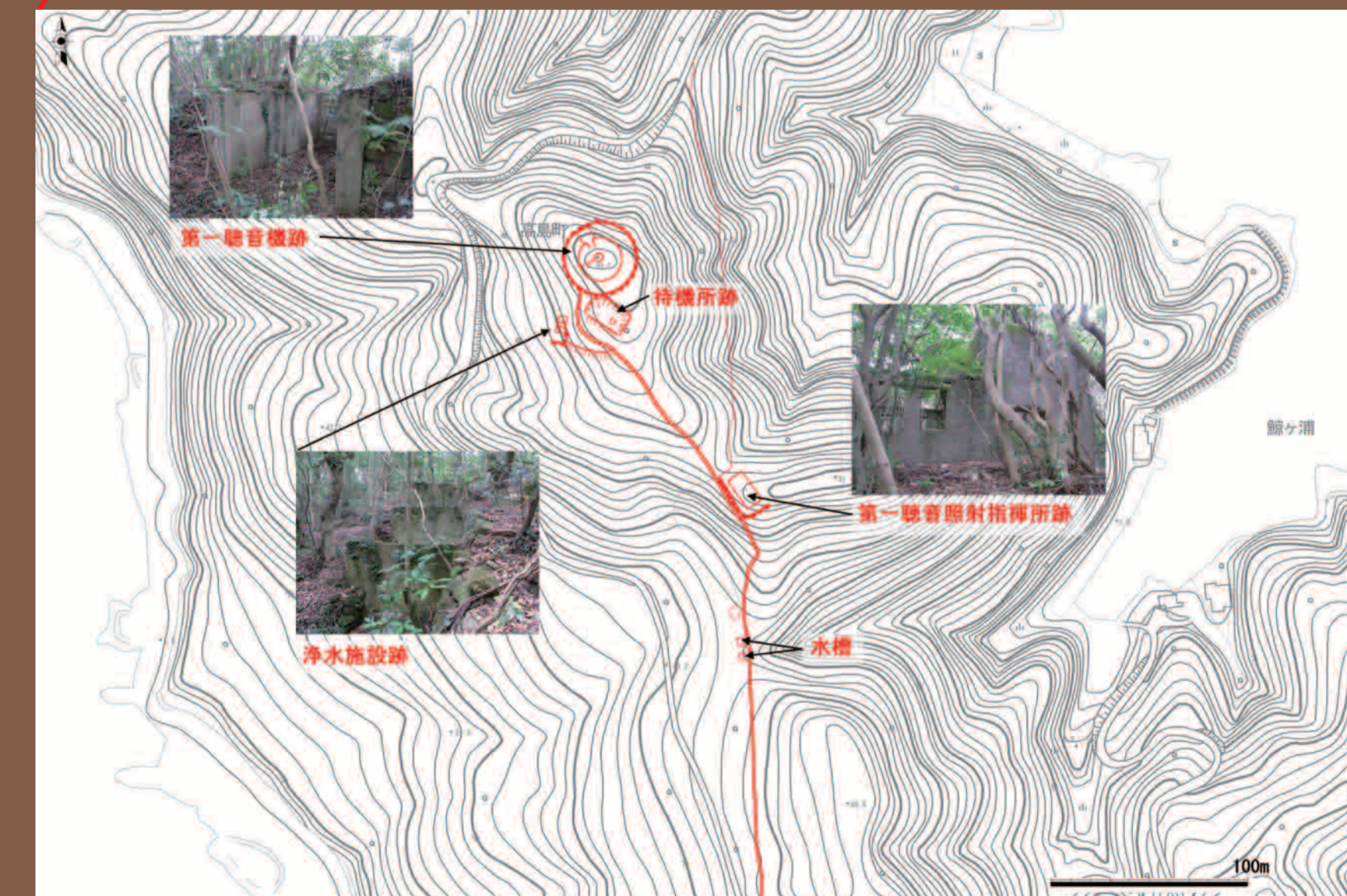
高島番岳高射砲台第一聴音照射所施設配置図
