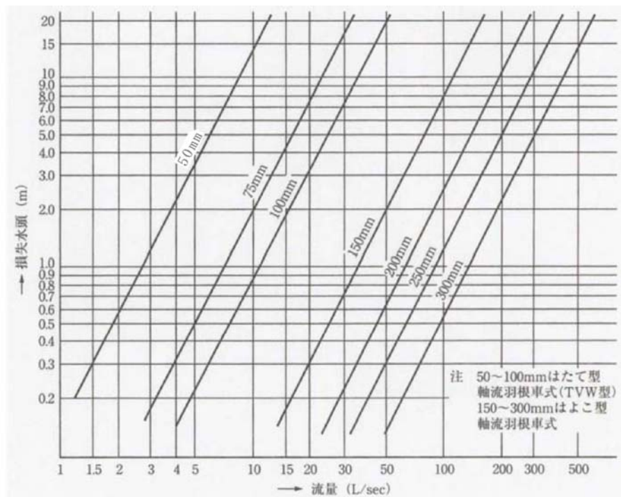
図 4-5 メーター口径の標準使用水量に対応する損失水頭
