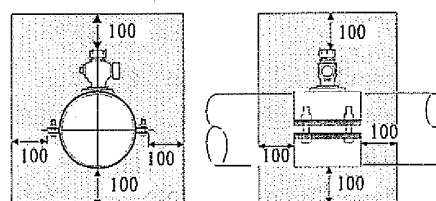
分水栓撤去工事の保護コンクリート
