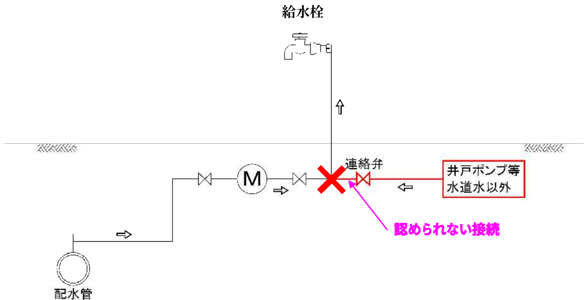
図 2-2 クロスコネクション（誤接合）の例
