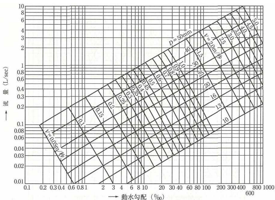
図 4-2 ウェストン公式流量図
