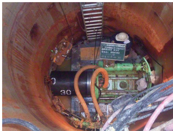
【推進工法による工事】
