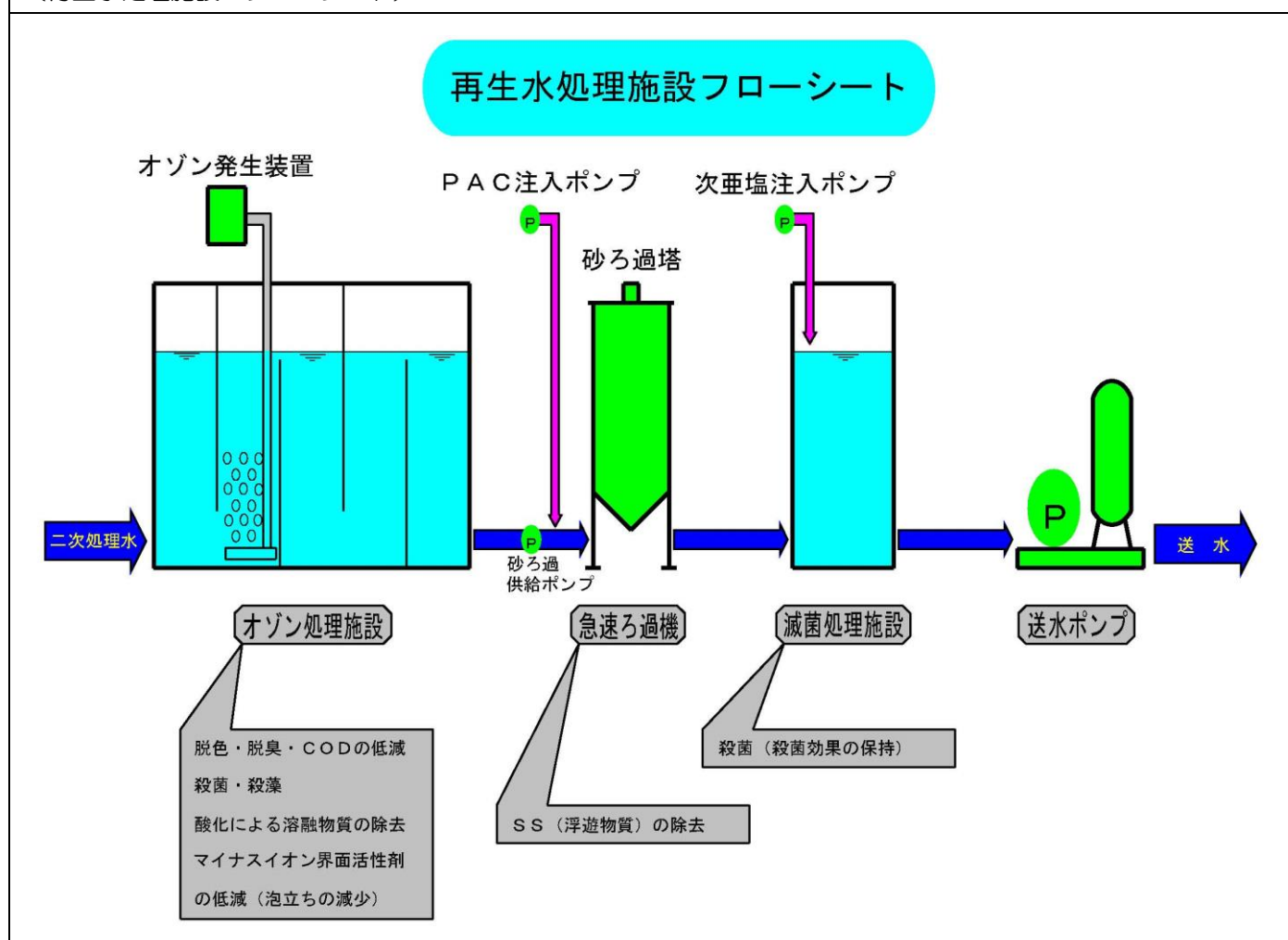
(再生水処理施設 フローシート)
