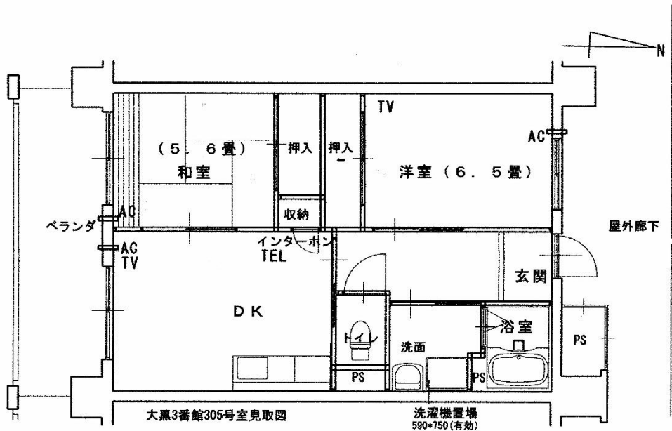
【間取り図】
