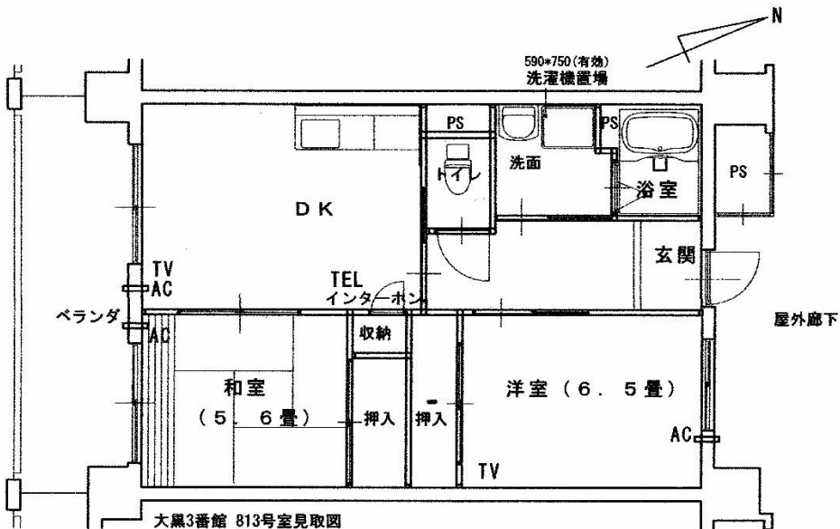
【間取り図】
