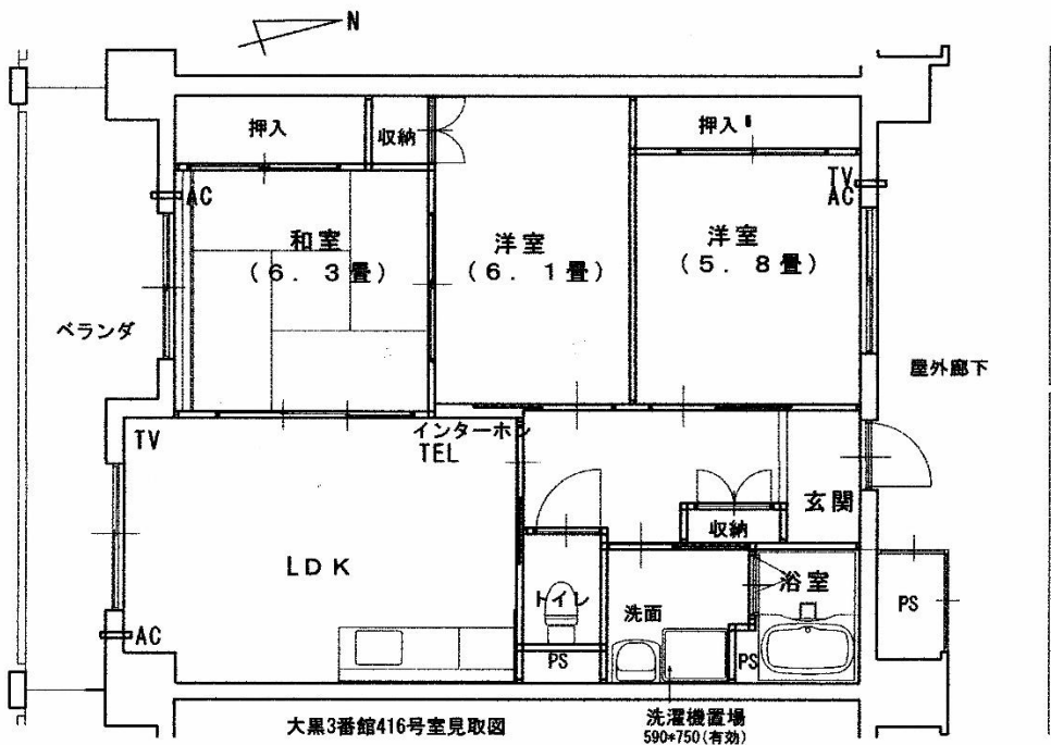
【間取り図】
