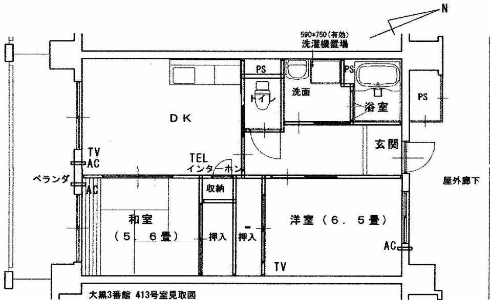
【間取り図】
