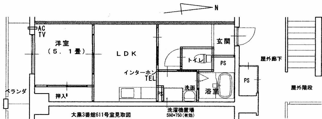
【間取り図】
