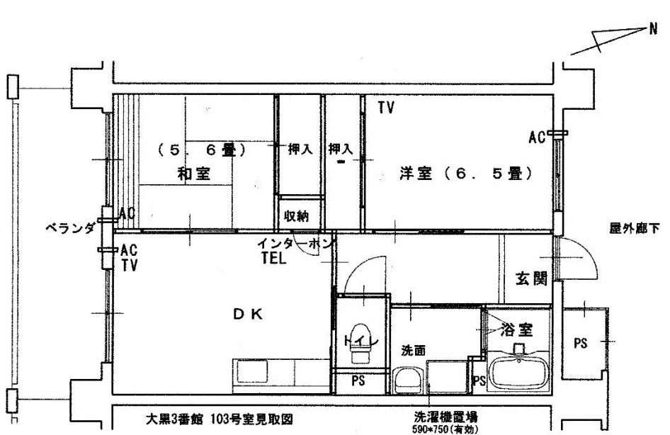
【間取り図】
