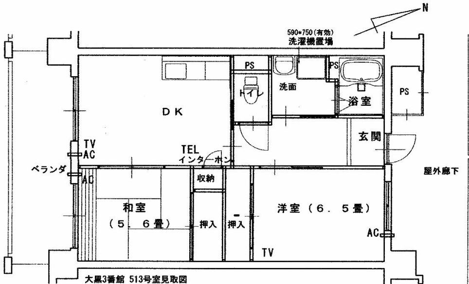
【間取り図】
