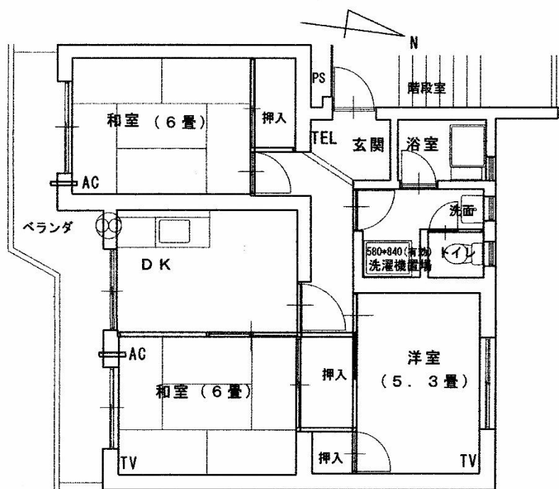
柚木第2住宅2棟205号見取図
