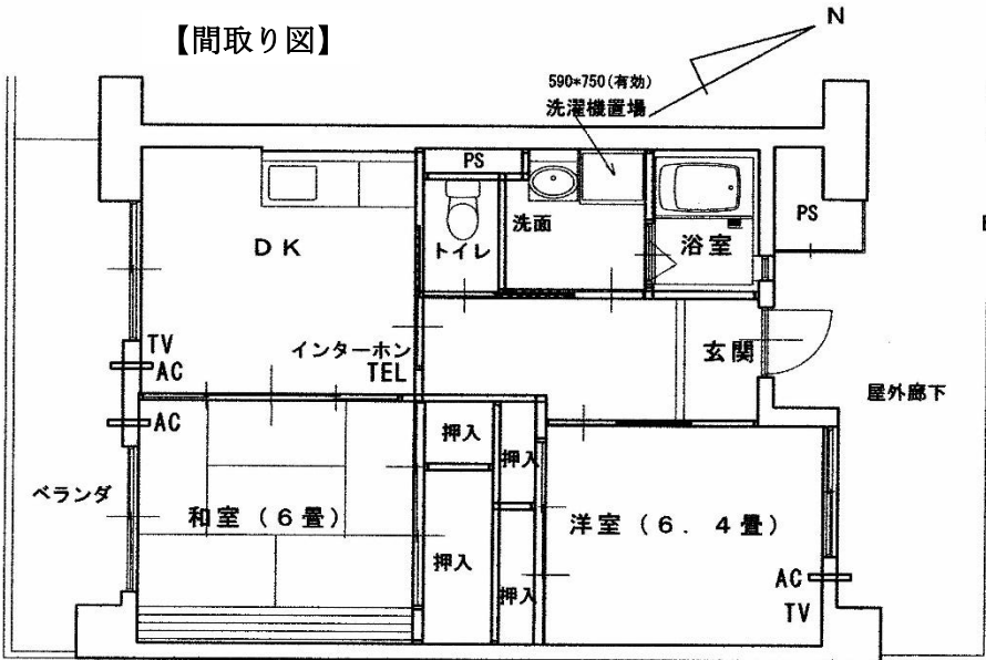
桜木2番館501号室見取図
