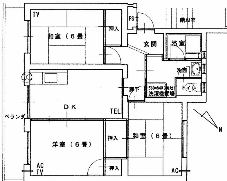
黒岩84棟305号室見取図
