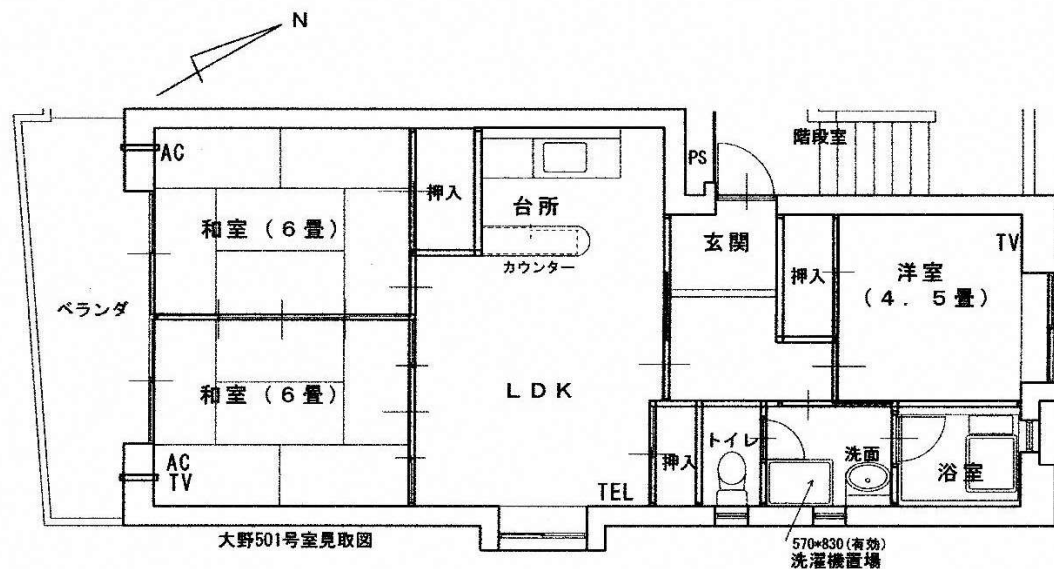
【間取り図】
