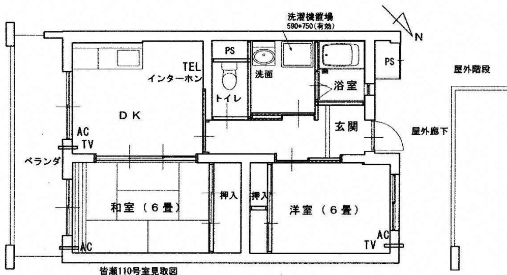
【間取り図】
